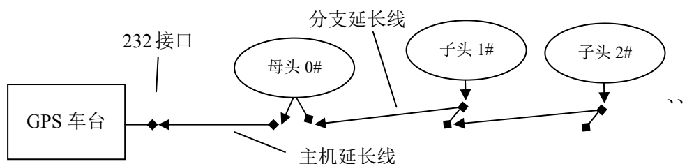
图中 → 代表有锁舌端， ← 代表相对的另一插头端。
