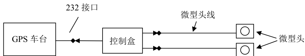
微型头和专用控制盒配套，微型头线一般长 3 米，加长有 5 米、8 米规格。
